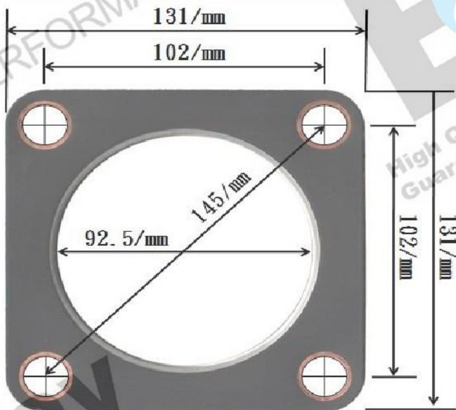
螺絲孔徑:15/mm 厚度:1.8/mm YANMAR MARINE 6EY17W 原廠號碼:133644-18710 品名:渦輪增壓器墊片*1(進氣接頭) 材質:二硫化鉬-1.8/mm
