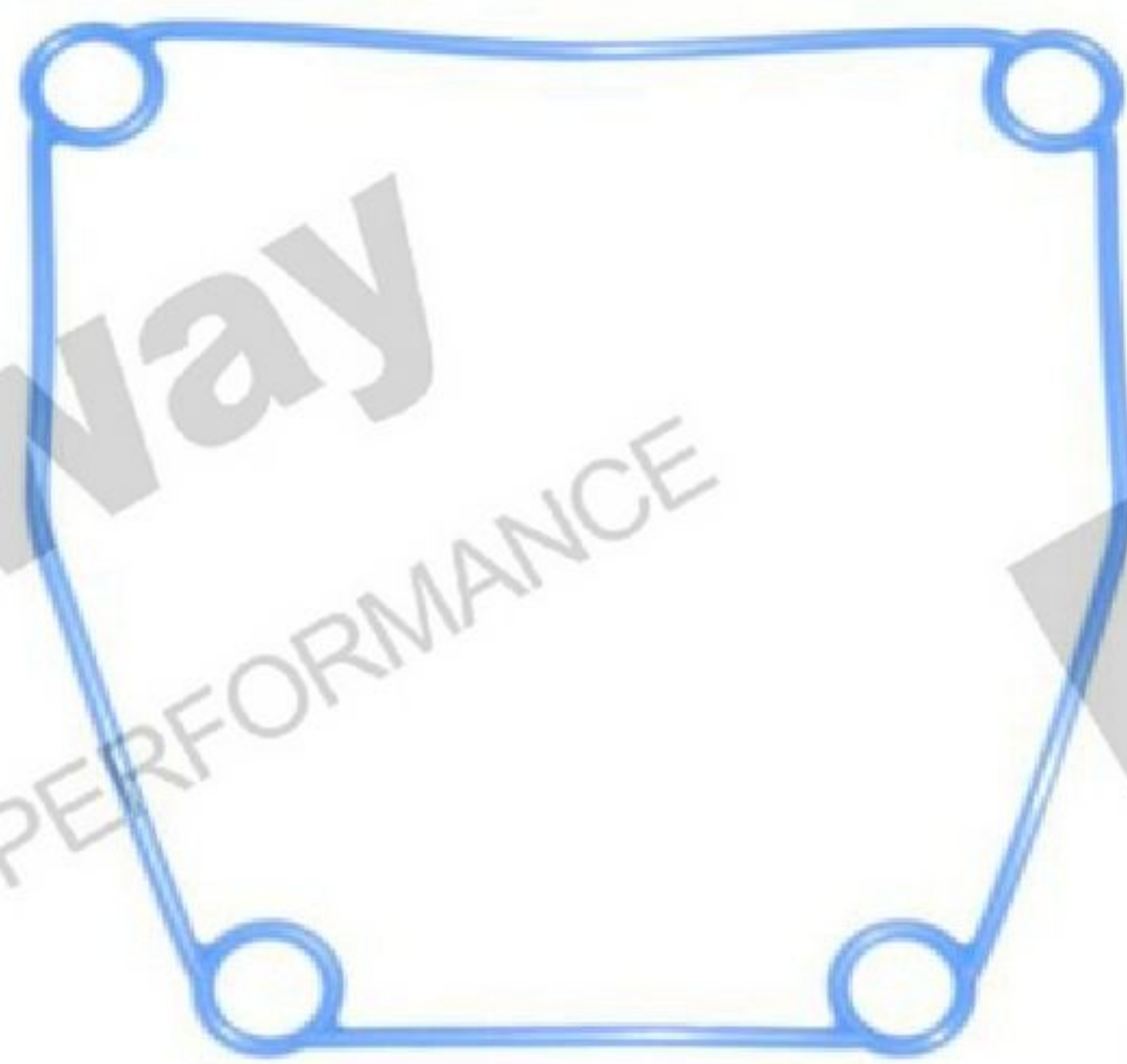
YANMAR MARINE 6EY17W 原廠號碼:140695-01470 品名:風門蓋/側蓋橡皮(*5)非操作面/飛輪面 材質:ACM(藍色)
